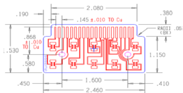
图 4: 安装有 XLamp XB-D LED 封装的 MCPCB 板
