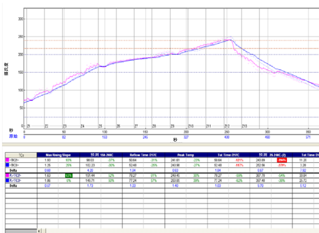
图 6: 无铅 (SAC) 焊料回流温度曲线。峰值温度: 240.98 °C, 维持高于 217 °C 的时间: 52.48 秒
