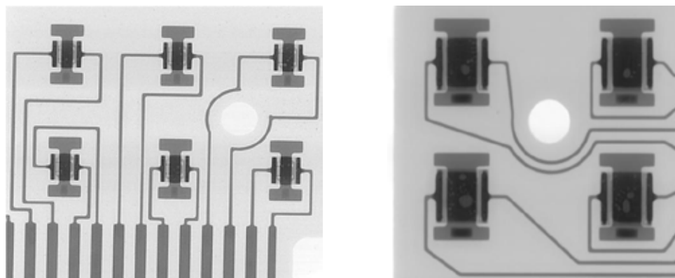
图 8: PCB 上 XP-G LED 封装（左）和 XM-L HVW LED 封装（右）在焊接空洞 < 30% 时的 X 射线成像
