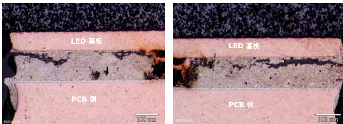
图 14: 热冲击测试后 PCB 与 XLamp XP-G LED 封装间的焊点
