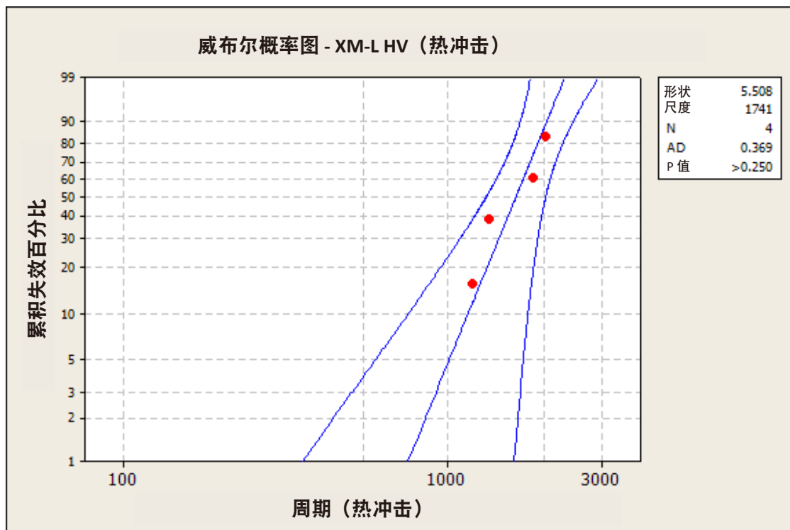
图 11: XM-L HVW 热冲击测试, -40 °C 到 125 °C, 最多 2000 个周期
