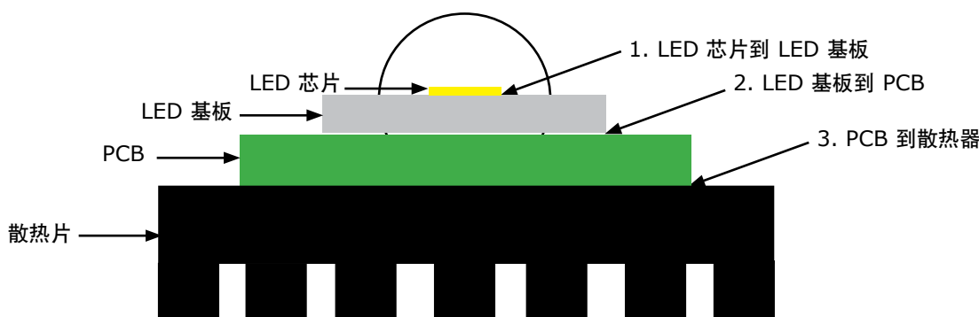
图 1: 确保热量从 LED 结点传递到散热器的重要焊点
