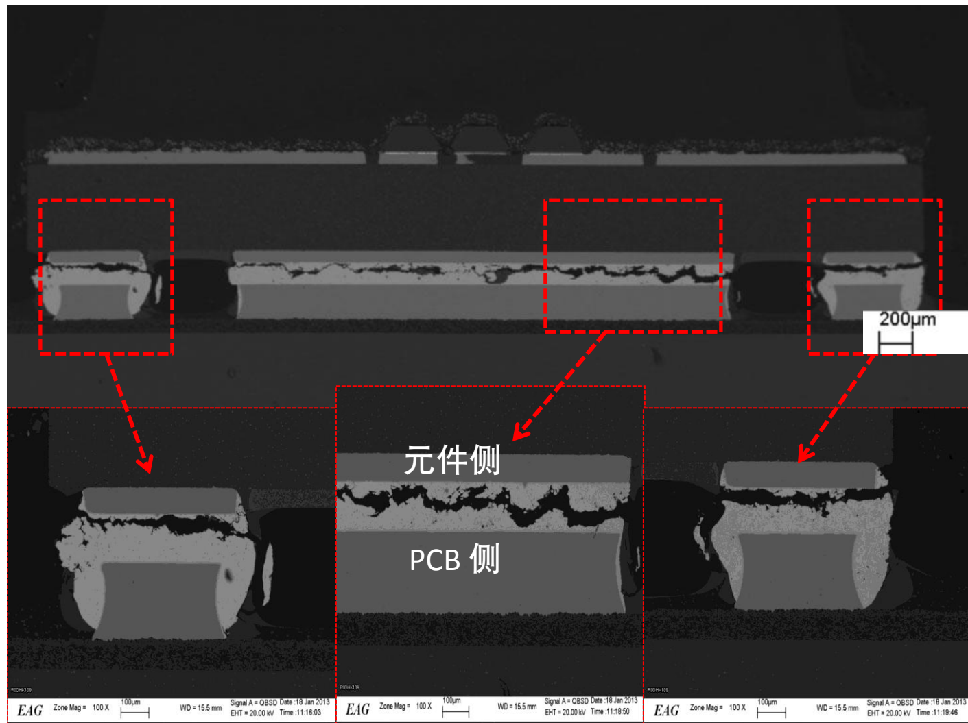
图 18: 显示热冲击测试后焊点裂纹的 XM-L HVW LED 封装横截面 SEM 显微图
