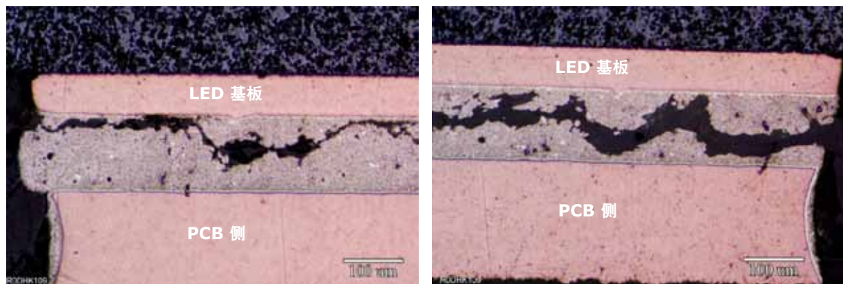
图 16: 热冲击测试后 PCB 与 XLamp XM-L HVW LED 封装间的焊点
