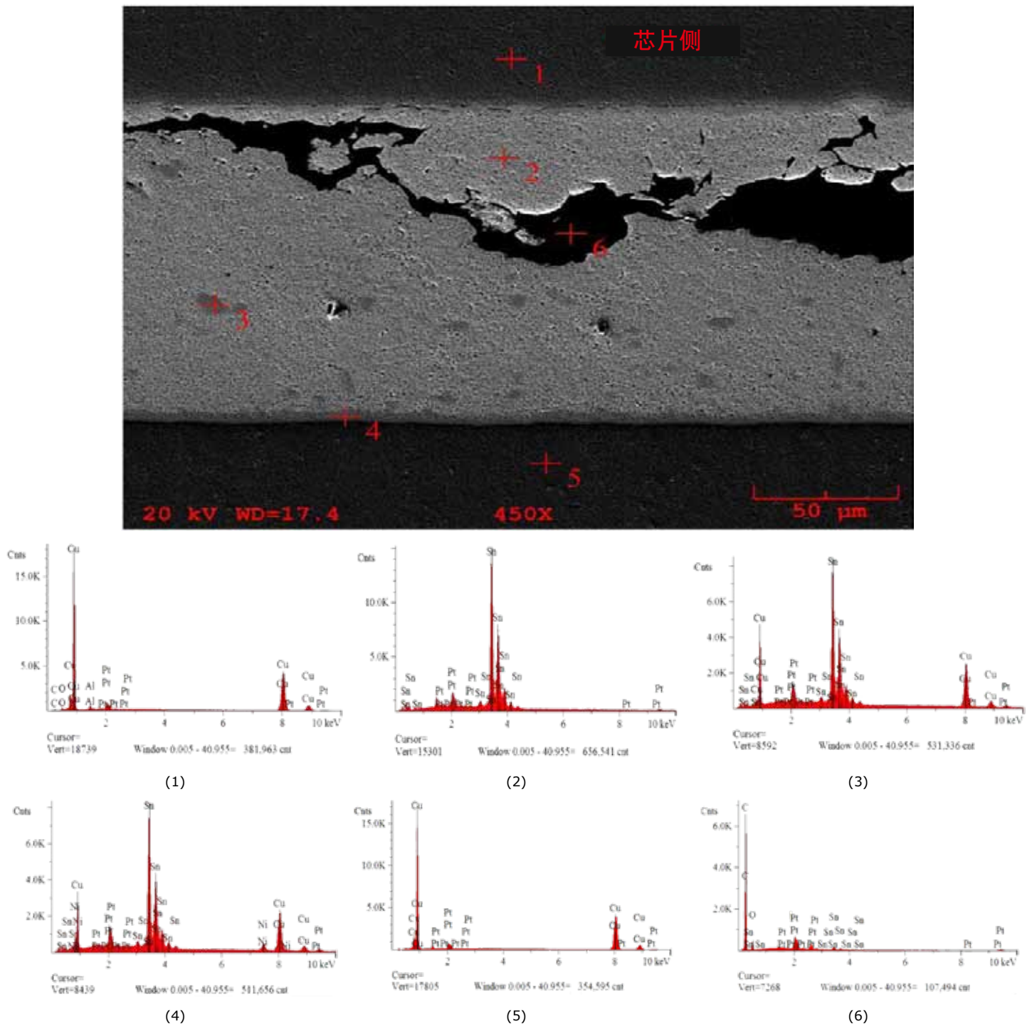
图 19: XM-L HVW 焊点 (顶部) 与 EDX 分析位置
