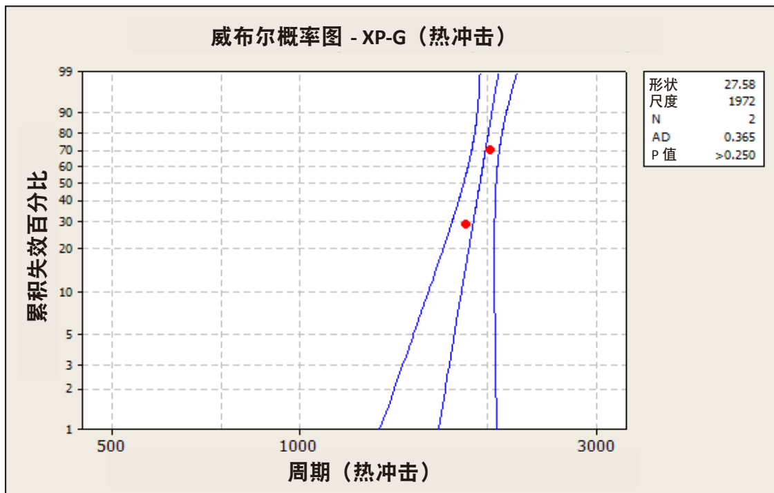
图 10: XP-G 热冲击测试, -40 °C 到 125 °C, 最多 2000 个周期
