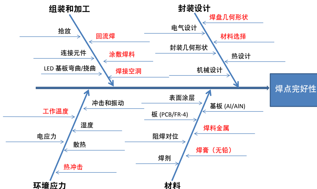
图 2: 通常会影响 LED 焊点完整性的因素
