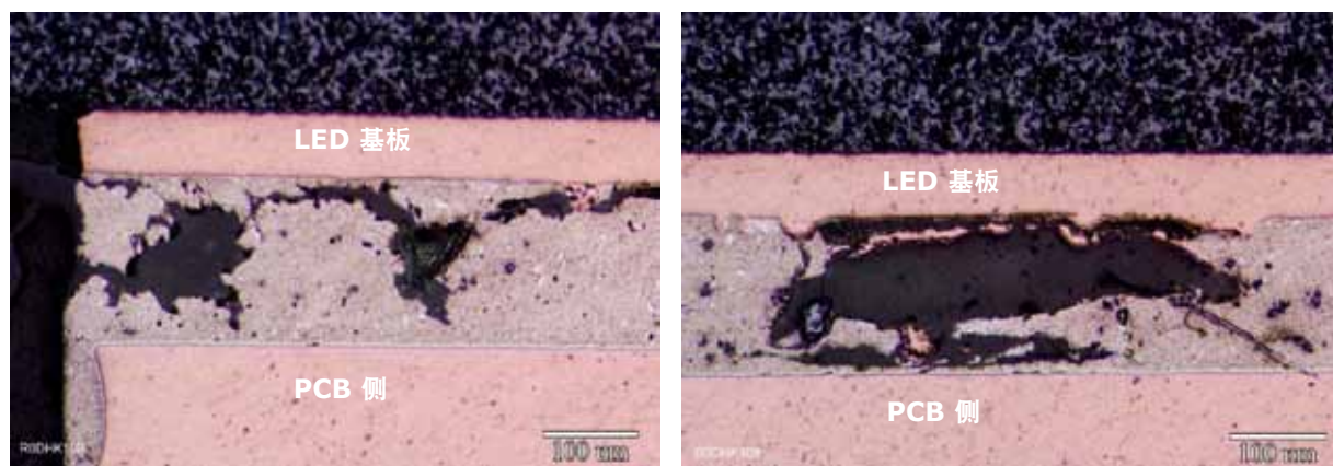
图 15: 热冲击测试后 PCB 与 XLamp XM-L LED 封装间的焊点回流焊后, XM-L LED 封装下方的空洞超过 50%。
