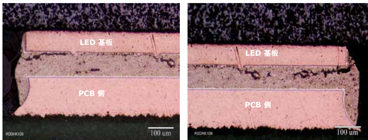
图 13: 热冲击测试后 PCB 与 XLamp XB-D LED 封装间的焊点
