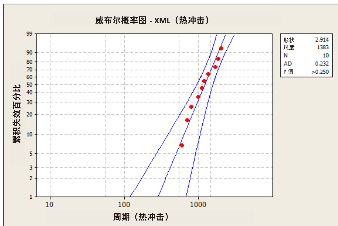
图 12: XM-L 热冲击测试, -40 °C 到 125 °C, 最多 2000 个周期
