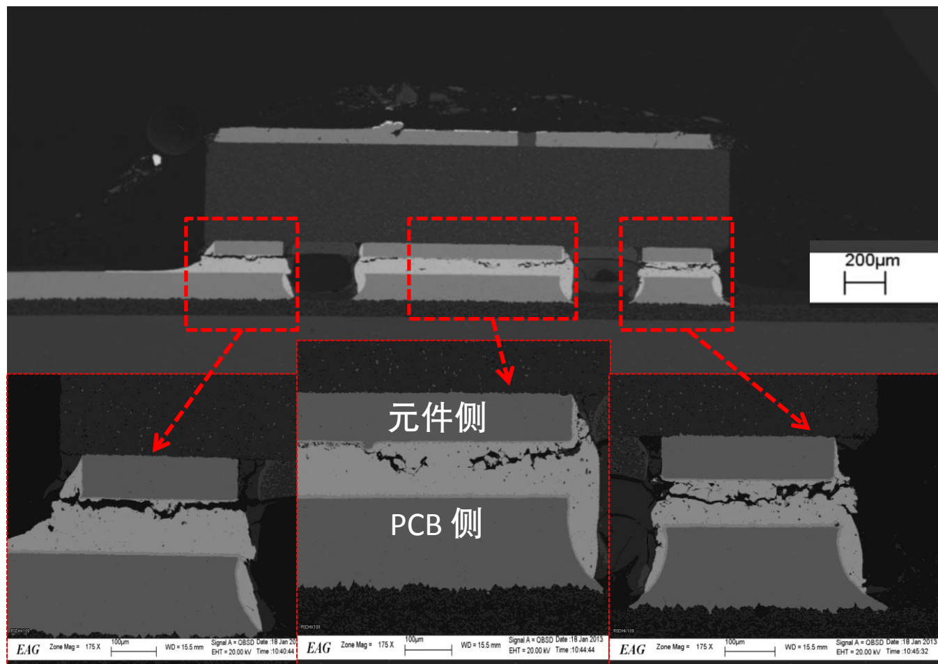
图 17: 显示热冲击测试后焊点裂纹的 XB-D LED 封装横截面 SEM 显微图
