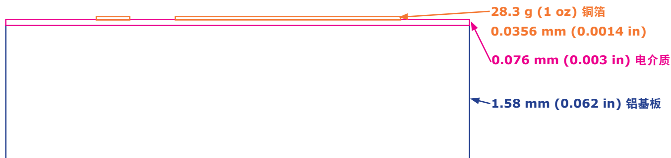
图 5: MCPCB 的横截面
