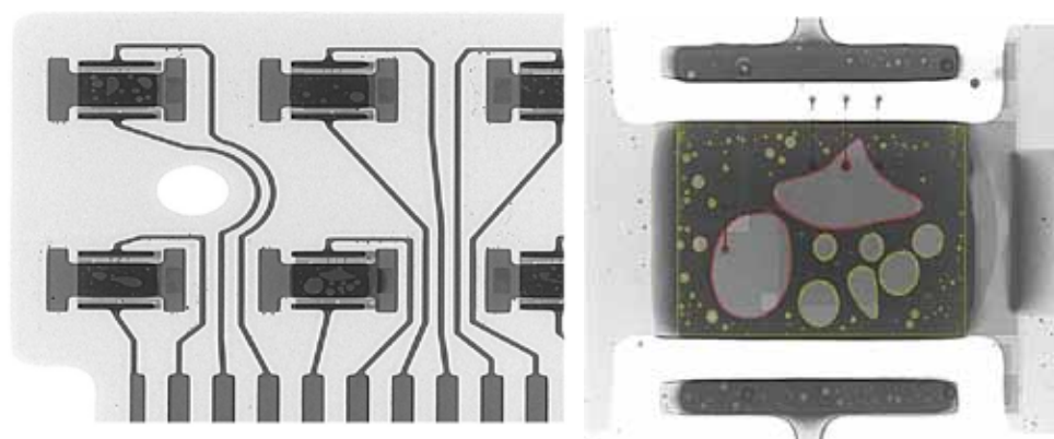
图 9: PCB 上 XM-L LED 封装在出现大量空洞 (> 50%) 时的 X 射线成像
